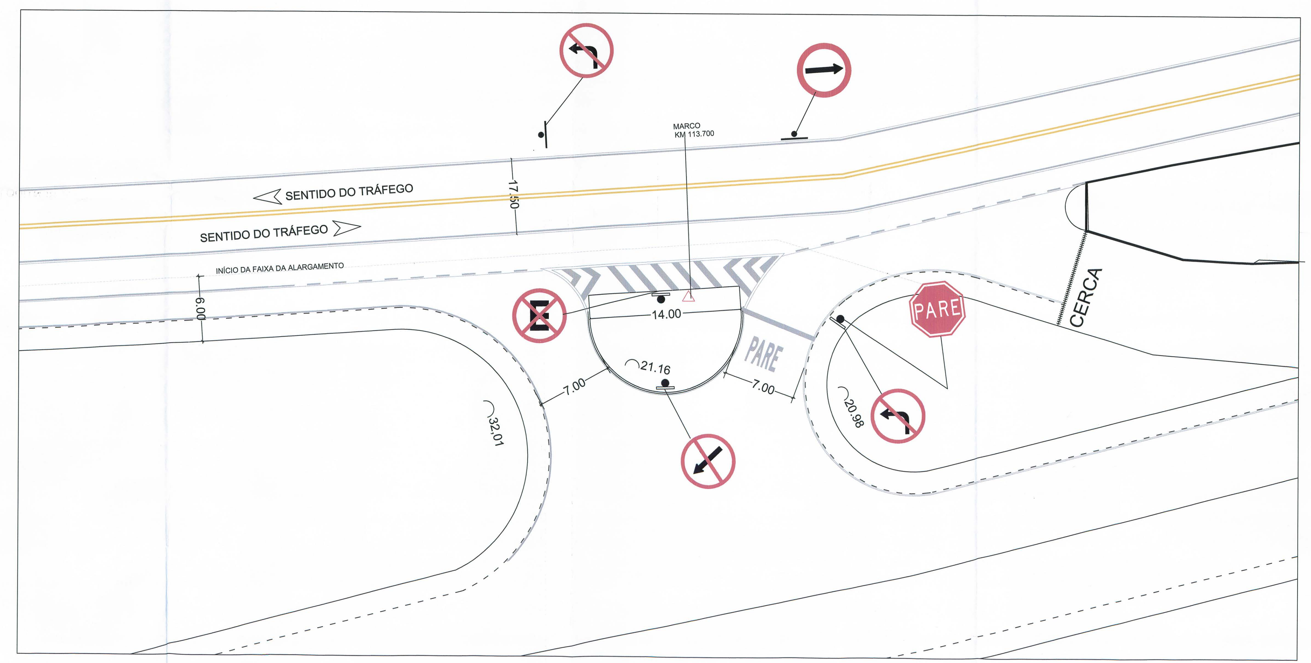
DETALHE AMPLIADO DO ACESSO esc. 1:200
